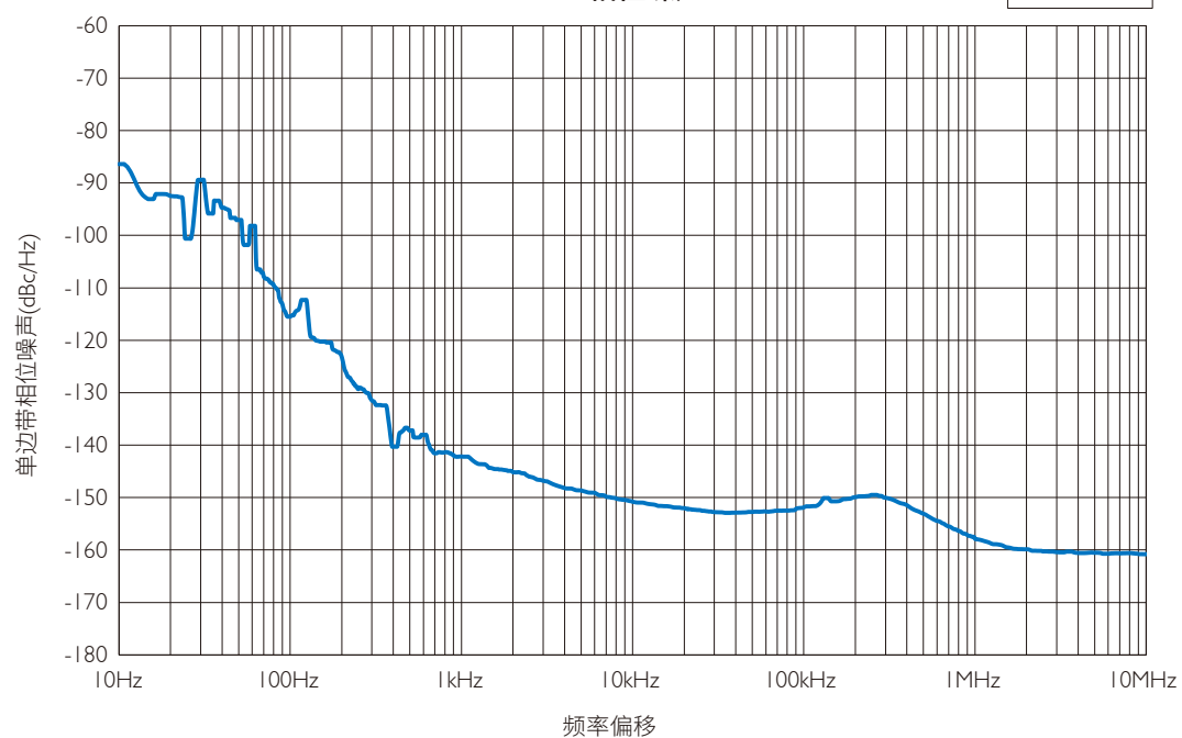
1GHz相位噪声
